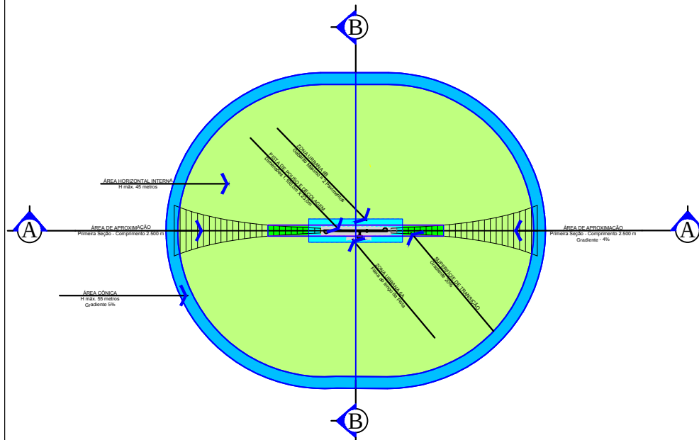
ÁREA DE PROTEÇÃO DO AERODROMO HELMUTH BAUNGARTEN PORTARIA nº 256/GC5/2011 Código da Pista 2 - Visual
