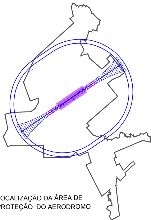
ÁREA DE PROTEÇÃO DO AERODROMO HELMUTH BAUNGARTEN PORTARIA nº 256/GC5/2011 Código da Pista 2 - Visual
