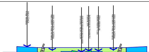
ÁREA DE PROTEÇÃO DO AERODROMO HELMUTH BAUNGARTEN PORTARIA nº 256/GC5/2011 CORTE BB
